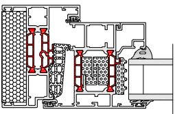
➤ 58BW FLUSH HI JAMB
