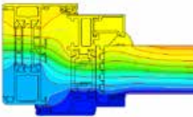
► 58BWST HI THERMAL PROFILE
