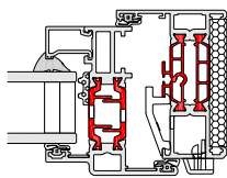
► 58BWST HI OPEN OUT CIL
